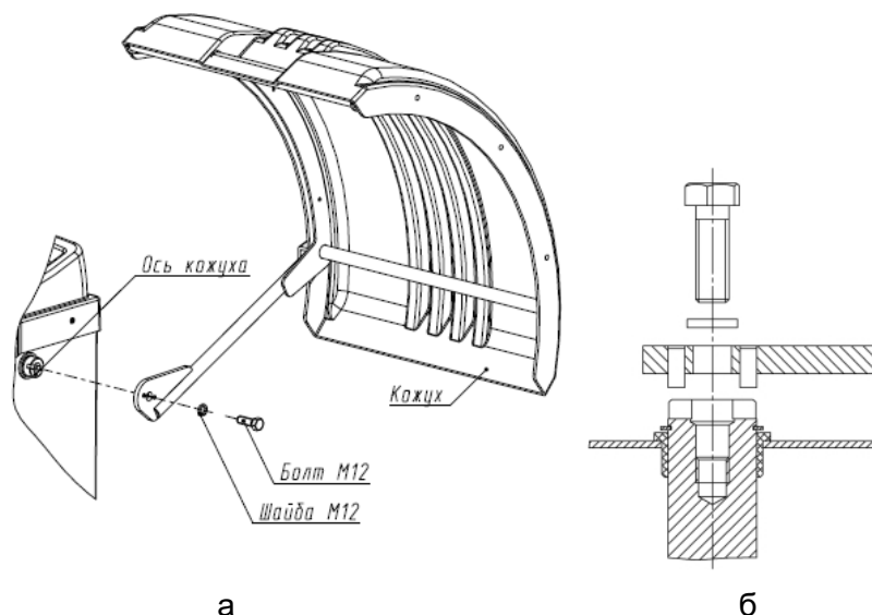
Рисунок 4.3 – Установка кожуха
